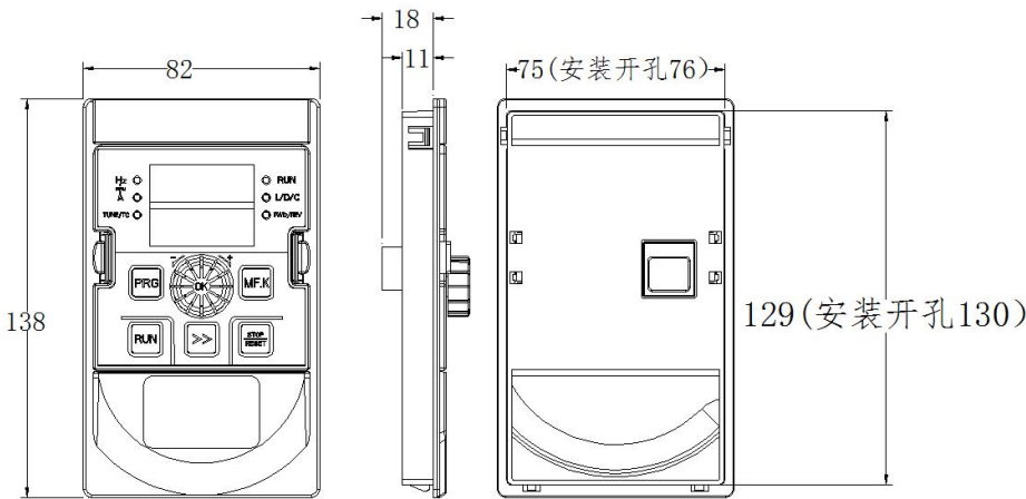
图 2-8. 1 外引键盘带托盘安装尺寸图
