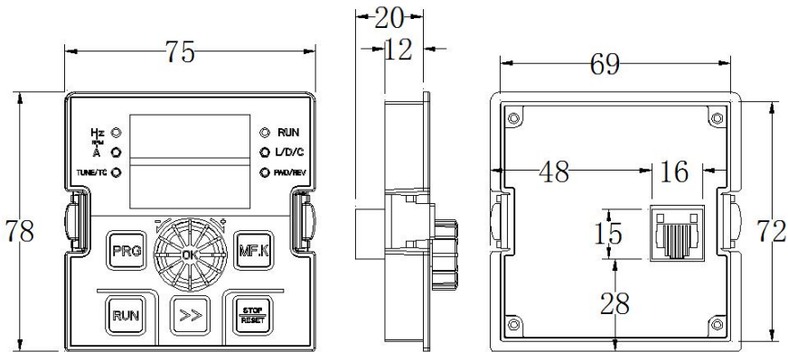
图 2-9.1 外引键盘不带托盘安装尺寸图
