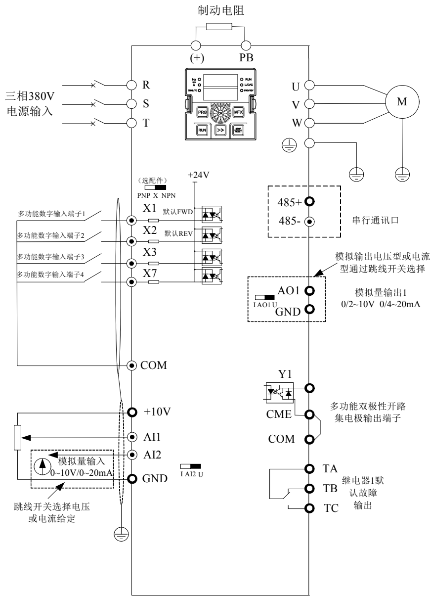
图3-1. 三相380V 2.2kW（4T:380V）及单相220V（2S）1.5kW(输入接L N或R T)以下变频器接线图
